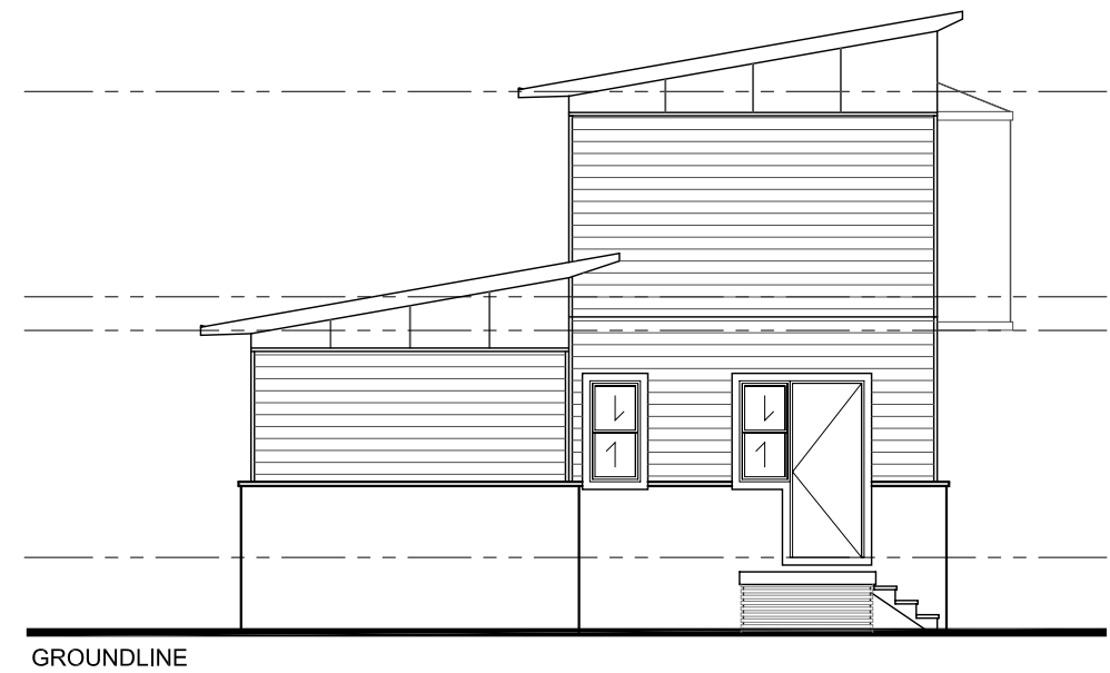
ELEVATION B
